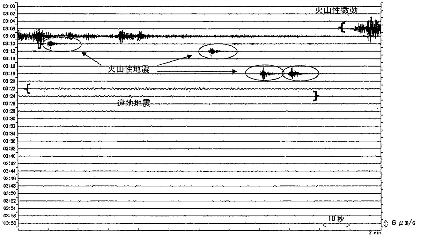
図 3 御嶽山 微動及び地震の発生状況
