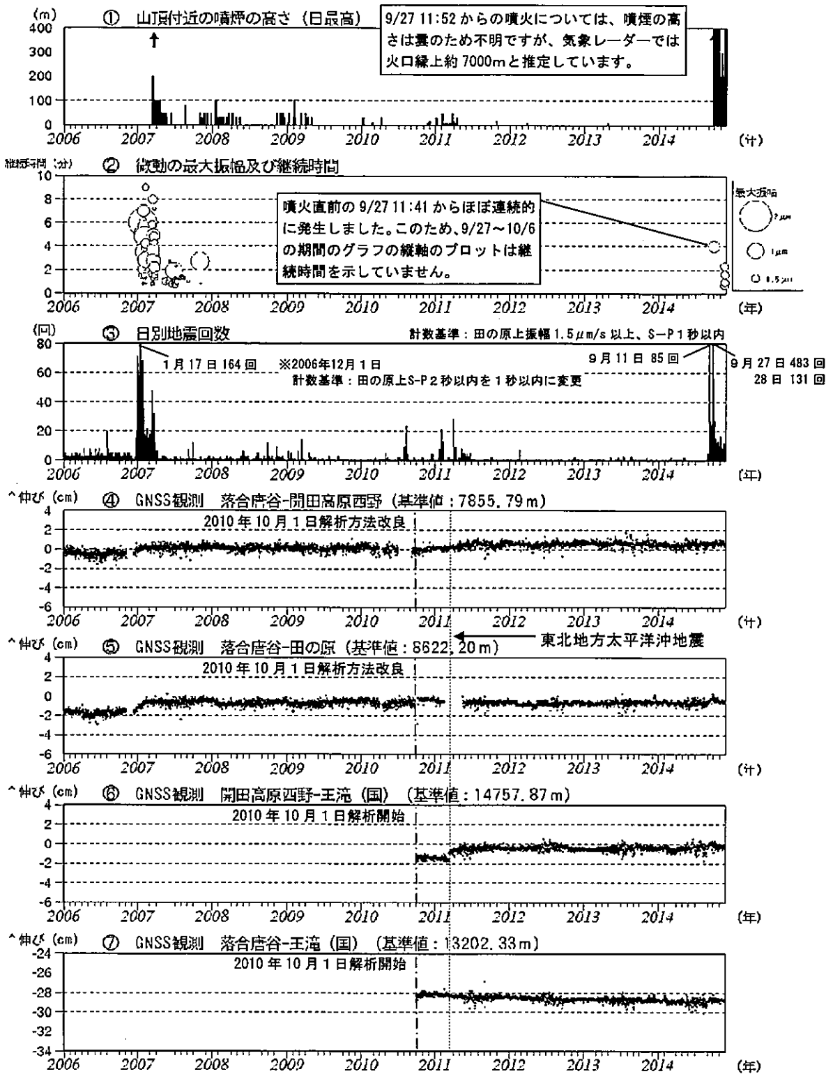
図5 御嶽山 長期間の火山活動経過図（2006年1月1日～2014年11月30日）
