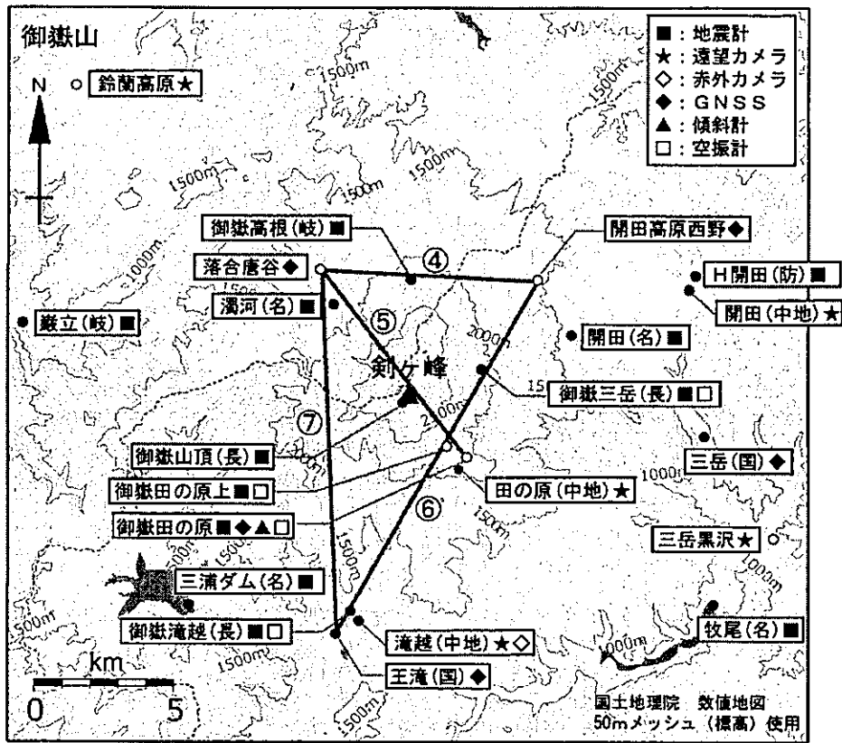
図9 御嶽山 観測点配置図
