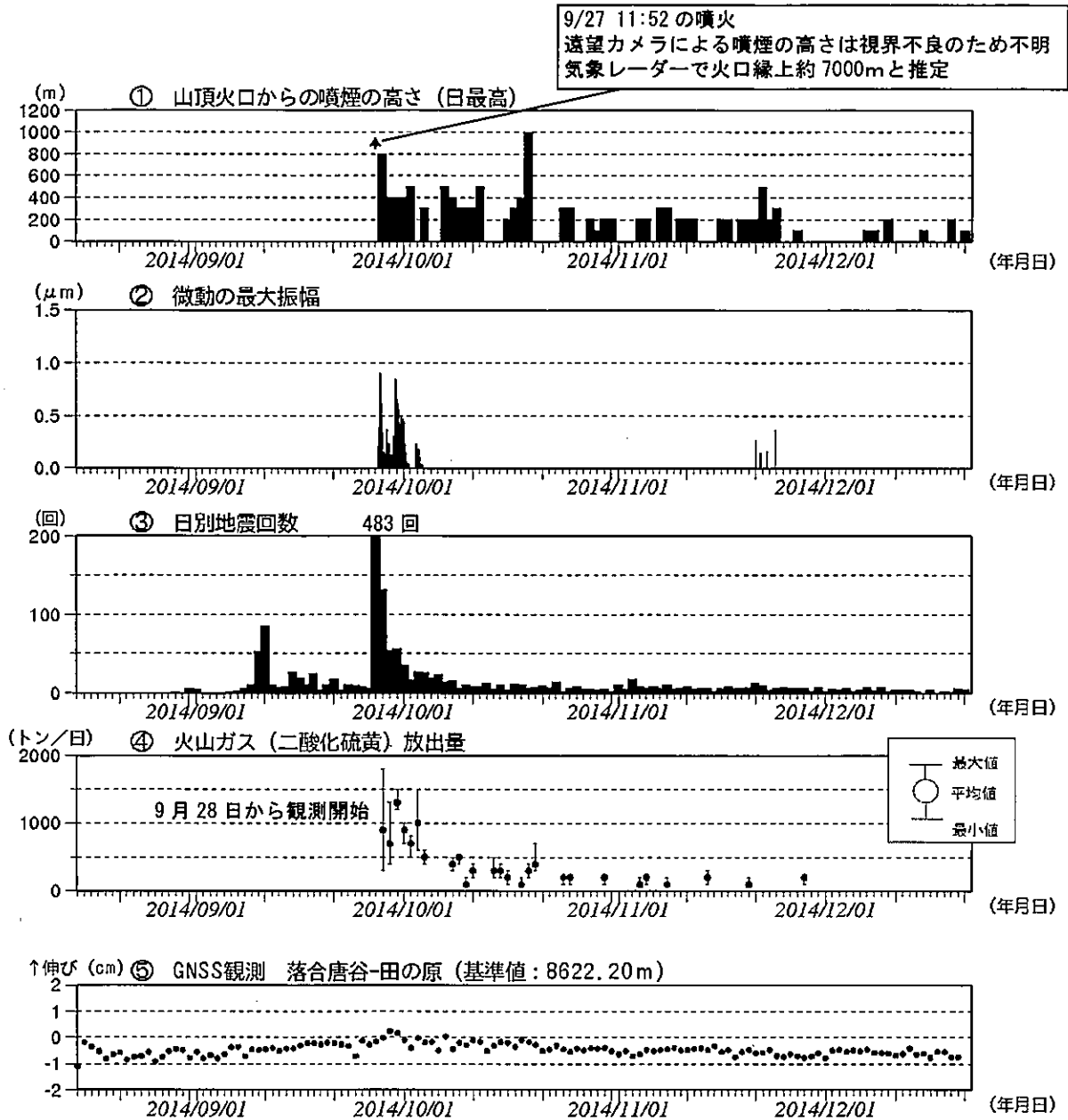
図 2 御嶽山 日別活動状況 (2014 年 8 月 15 日~12 月 21 日 (速報値含む))
