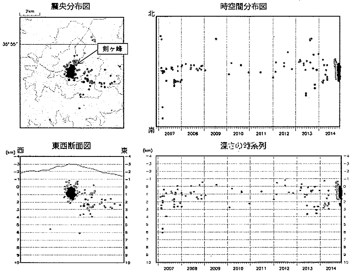
図2 御嶽山 震源分布図 (2006年12月1日~2014年11月30日)
