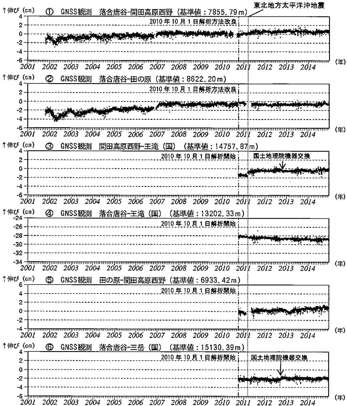
図3 御嶽山 GNSS 連続観測による基線長の長期変化 (2001 年 1 月 1 日~2014 年 12 月 20 日)
