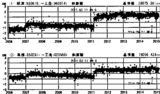
基線変化グラフ
