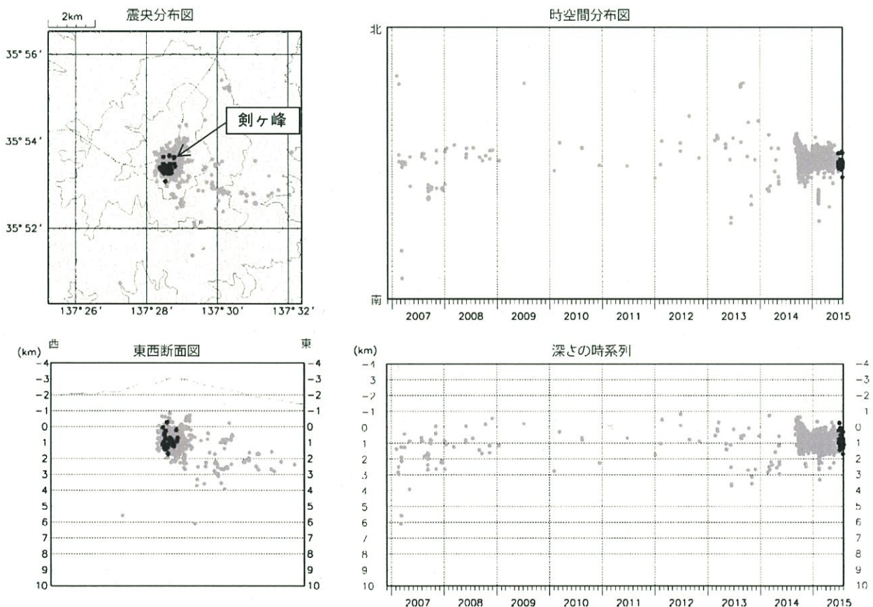
図 2 御嶽山 震源分布図（2006 年 12 月 1 日～2015 年 7 月 31 日）
