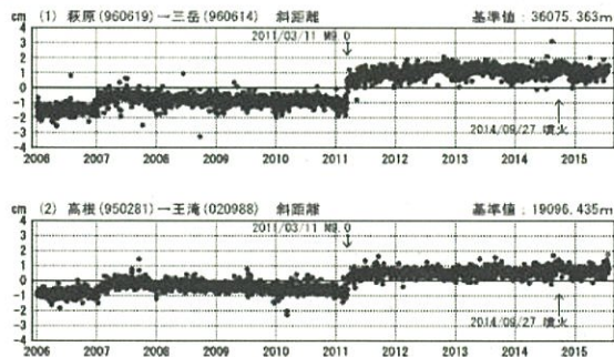
図 8 御嶽山 国土地理院による GNSS 基線変化グラフ 4)
