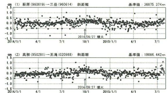
図 8 御嶽山 国土地理院による GNSS 基線変化グラフ 4)
