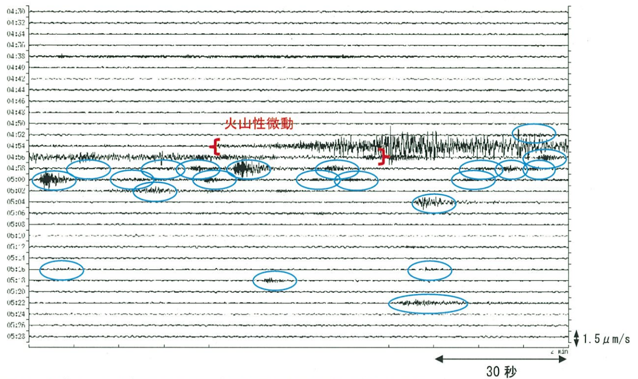
図3 御嶽山 火山性微動発生前後の地震の発生状況（青丸は地震）
