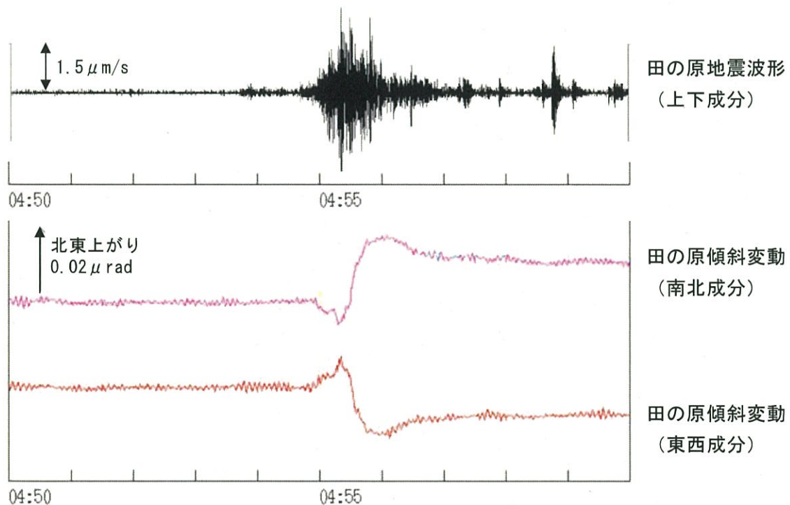
図4 御嶽山 火山性微動発生時の震動データ及び傾斜データ（秒値）の状況
